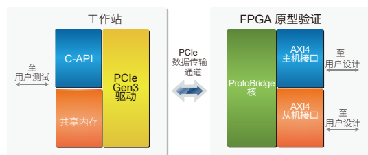
ProtoBridge AXI 架构
